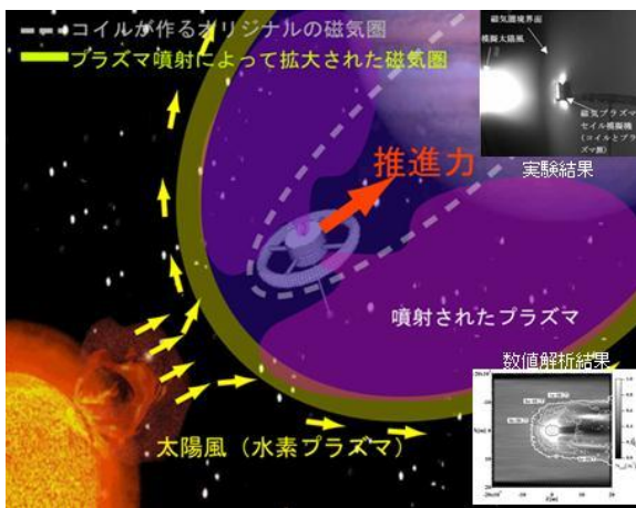
図1 磁気プラズマセイルの概要図および実験、数値解析結果
